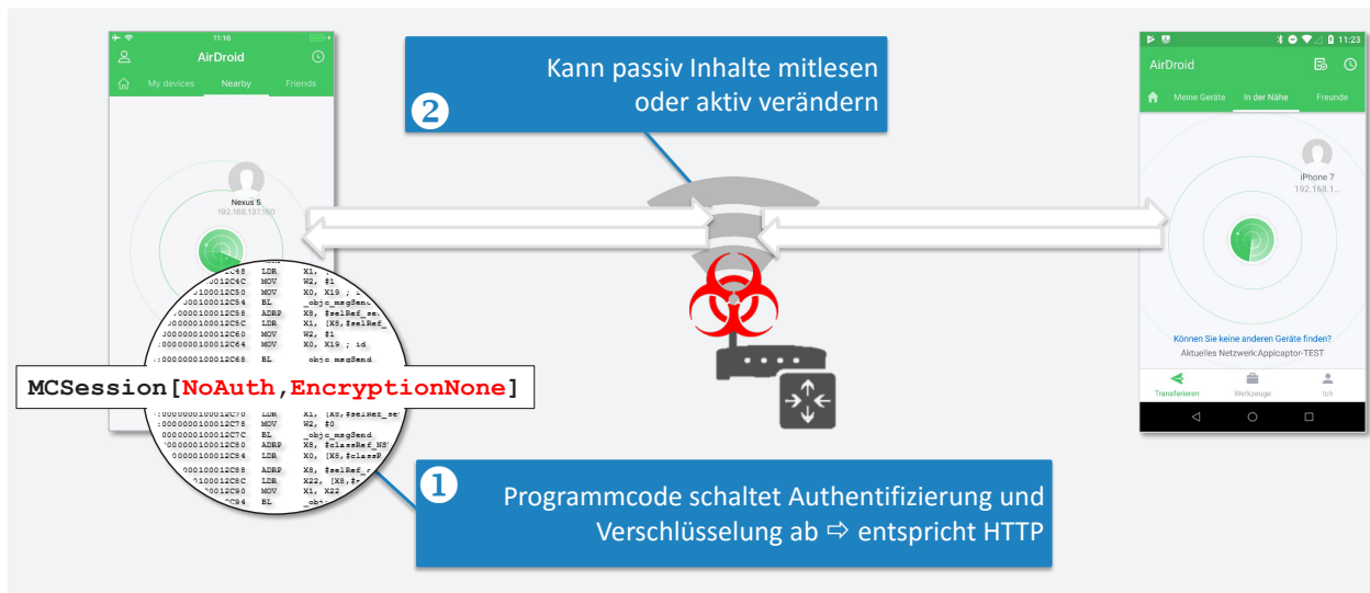
Abbildung 5: Schlechte / Fehlende Kryptographie: Gefährdung von Unternehmensdaten bei der Peer-To-Peer-Übertragung durch fehlende Verschlüsselung und Authentifizierung. Hier dargestellt an der AirDroid für iOS (Version 1.0.3)
