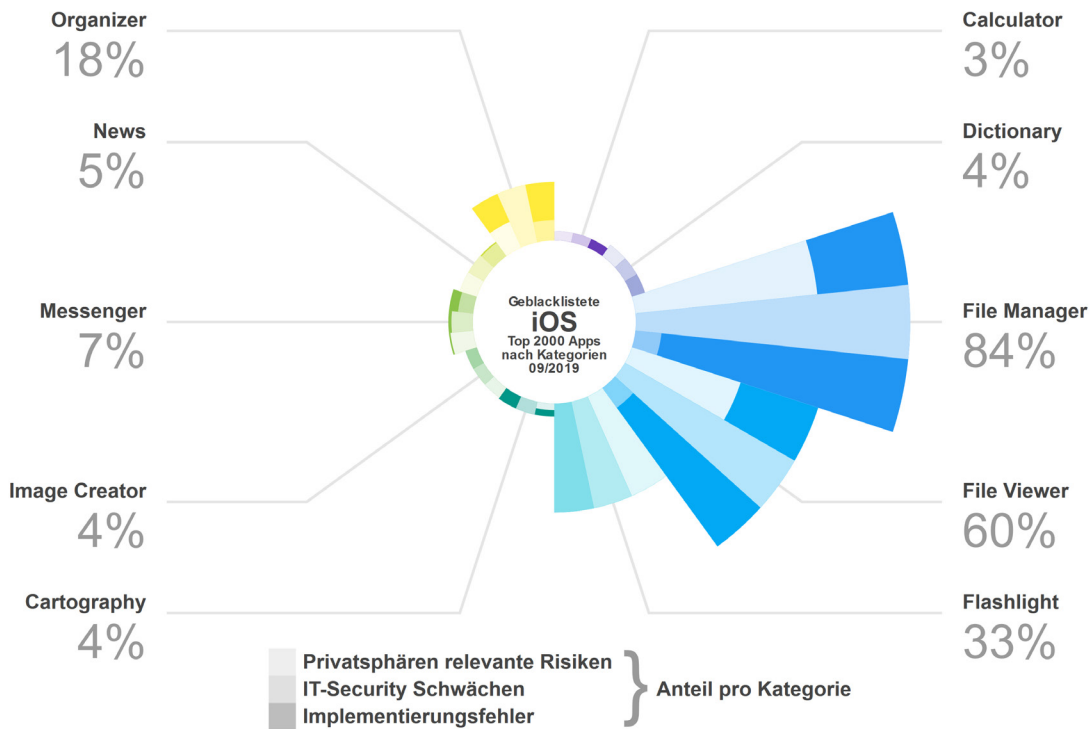
Abbildung 6: Anteil der geblocklisteten iOS-Apps je Funktionsklasse. Die Balken pro beispielhaft ausgewählter Funktionsklasse zeigen den jeweiligen Anteil der drei Risikoklassen. Bei den geblocklisteten 33% der Taschenlampen-Apps treffen jeweils alle Risiken zu. (Appcaptor, September 2019)
