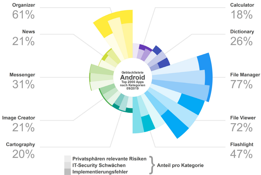
Abbildung 7: Anteil der geblocklisteten Android-Apps je Funktionsklasse. (Appcaptor, September 2019)
