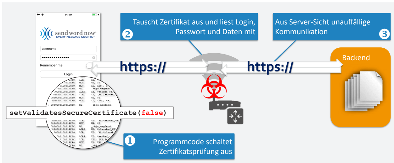
Abbildung 2: Altlasten aus der Entwicklungszeit: Gefährdung der Kommunikationssicherheit durch Abschalten der Server-Zertifikatsprüfung, die in der Produktivversion immer noch aktiv ist. Hier dargestellt mit der Send Word Now for iPhone App (Version 2.9.4)
