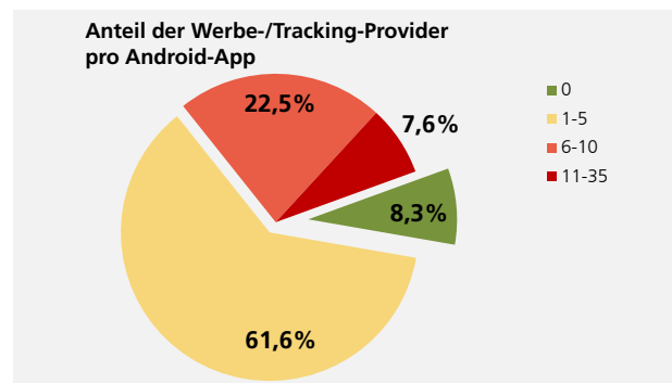
Abbildung 8: Anteil der Werbe- und Trackingnetzwerke pro iOS-/Android-App in den Top 2.000 der kostenlosen Apps der jeweiligen Plattform. In der Mehrzahl der Apps wurden bis zu 5 Werbe- und Trackingnetzwerke gefunden. Allerdings wurden auch Apps gefunden, die mit bis zu 57 solcher externen Dienstleister in Verbindung stehen. (Appcaptor, September 2019)
