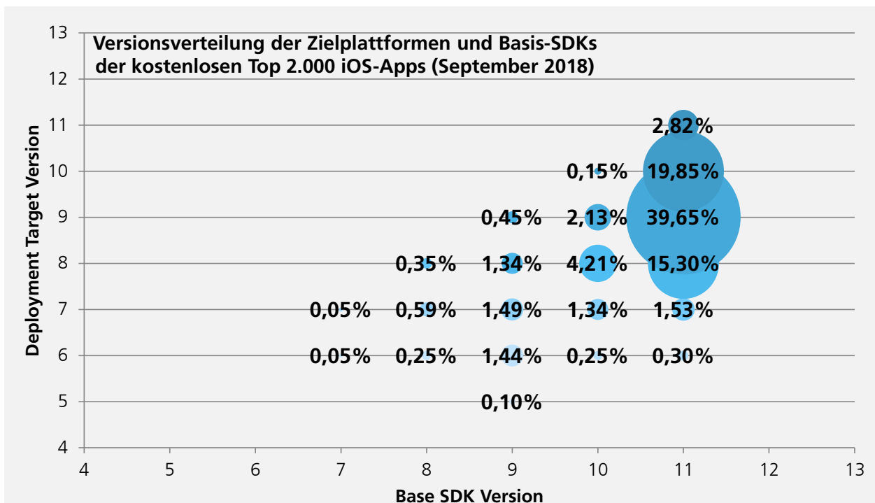
Abbildung 10: 20% der iOS-Apps wurden 2018 mit SDK-Versionen kleiner 11 erstellt, 2019 waren es nur noch 11%. (Appicaptor, September 2019)
