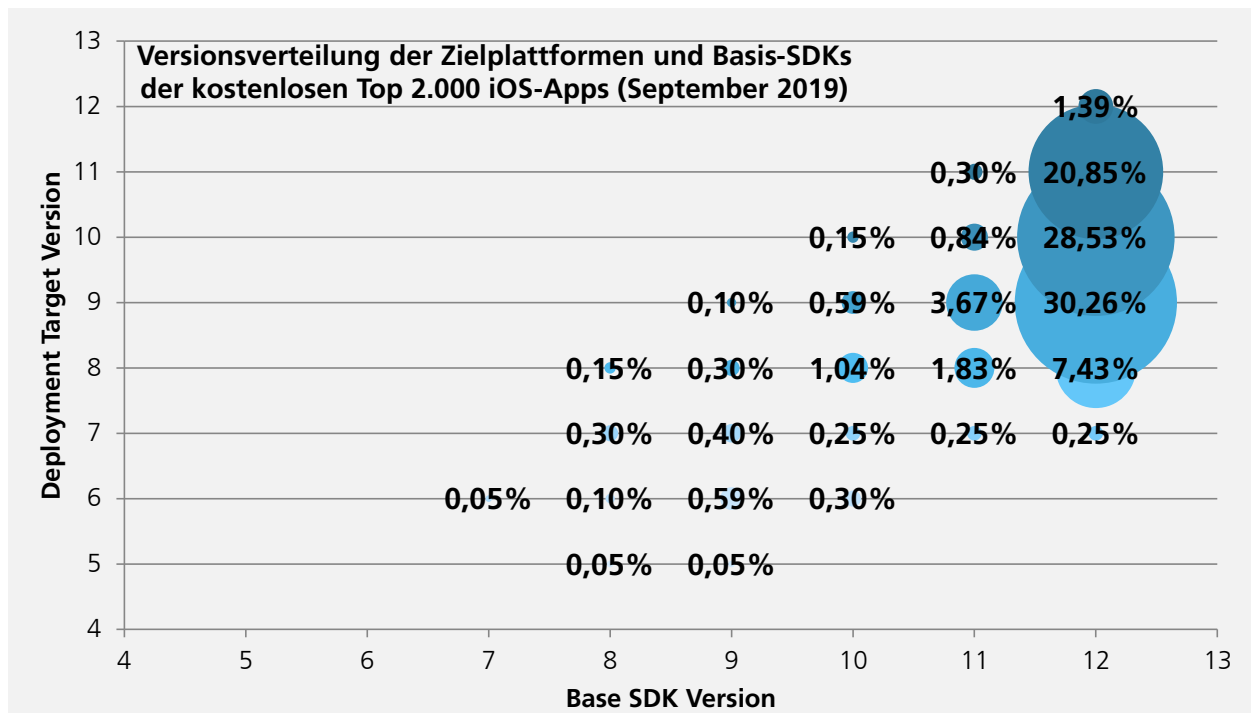
Abbildung 9: In 2019 ist die Anpassungsrate auf das aktuellste iOS SDK 12 sehr hoch. Nur 11% wurden mit einer vorherigen SDK Version erstellt (Appicaptor, September 2019)
