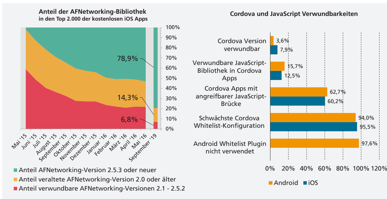
Abbildung 4: Auch nach der Veröffentlichung einer gravierenden Schwachstelle in der AFNetworking Bibliothek für iOS enthielten die kostenlosen Top 2.000 verwundbare Versionen. Nach über 4 Jahren sind immer noch 6,8% der genutzten AFNetworking-Versionen verwundbar. Auch in Hybrid-Apps werden noch verwundbare Versionen verwendet. (Appcaptor, September 2019)
