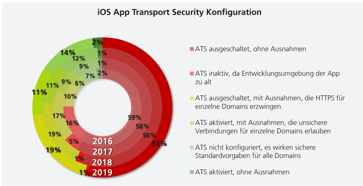
Abbildung 1: Aufteilung der Verwendung von App Transport Security bei den kostenlosen Top 2.000 iOS-Apps (Appcaptor, September 2019)
